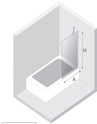
Opcja 1 Wspornik skośny
