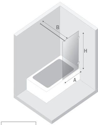
Opcja 2 Wspornik prostopadły
